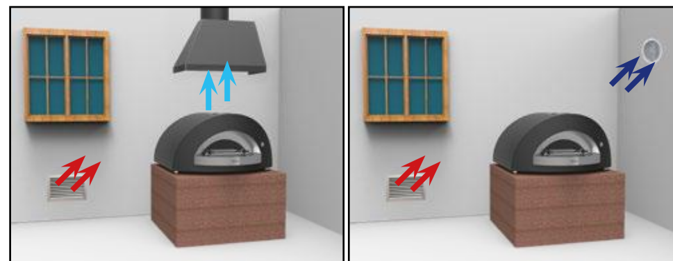
➔ VENTILAZIONE FORZATA - 1,72 m 3 /h x kW ➔ AERAZIONE FORZATA - 1,72 m 3 /h x kW
