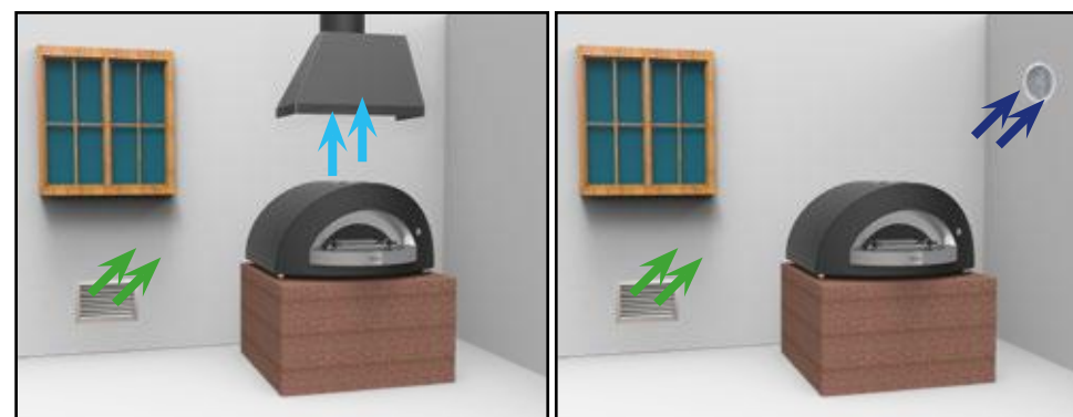
➔ VENTILAZIONE NATURALE - S=300cm 2 ➔ AERAZIONE FORZATA - 1,72 m 3 /h x kW
